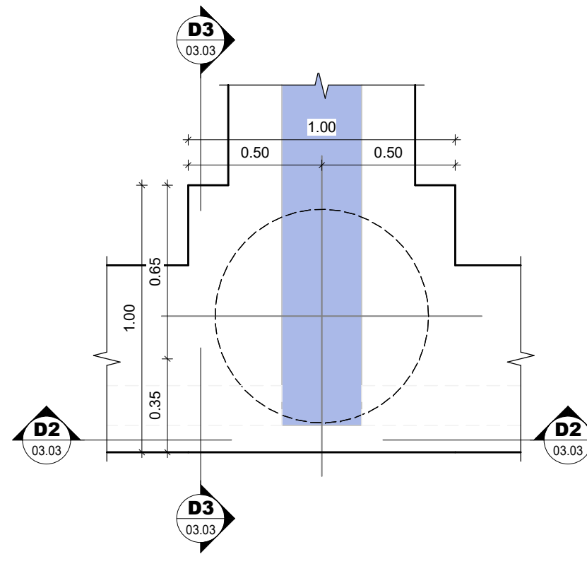
GEOMETRÍA TÍPICA DADOS TIPO 3 Y 4 Escala 1 : 20
