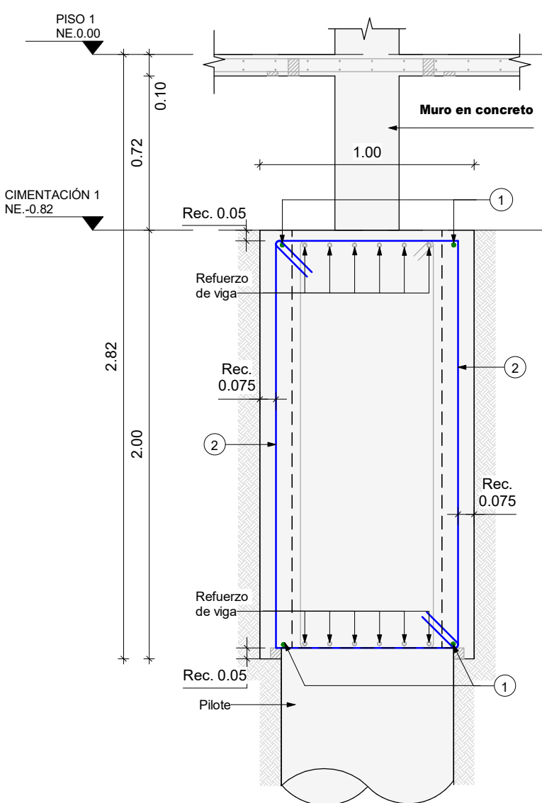
CORTE D1 Escala 1 : 25 DADO TIPO 1
