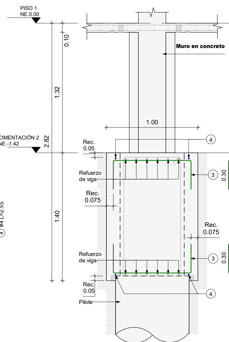
CORTE D2 Escala 1 : 25 DADO TIPO 2 Y 4
