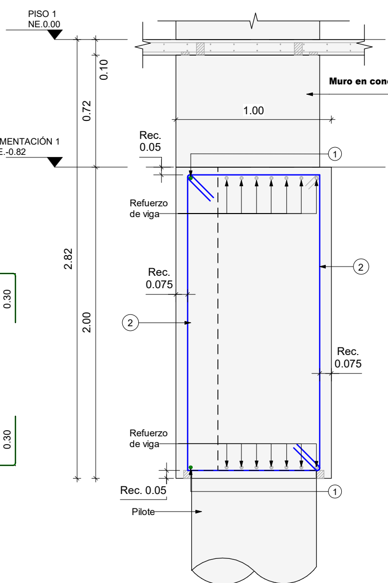
CORTE D3 Escala 1 : 25 DADO TIPO 3
