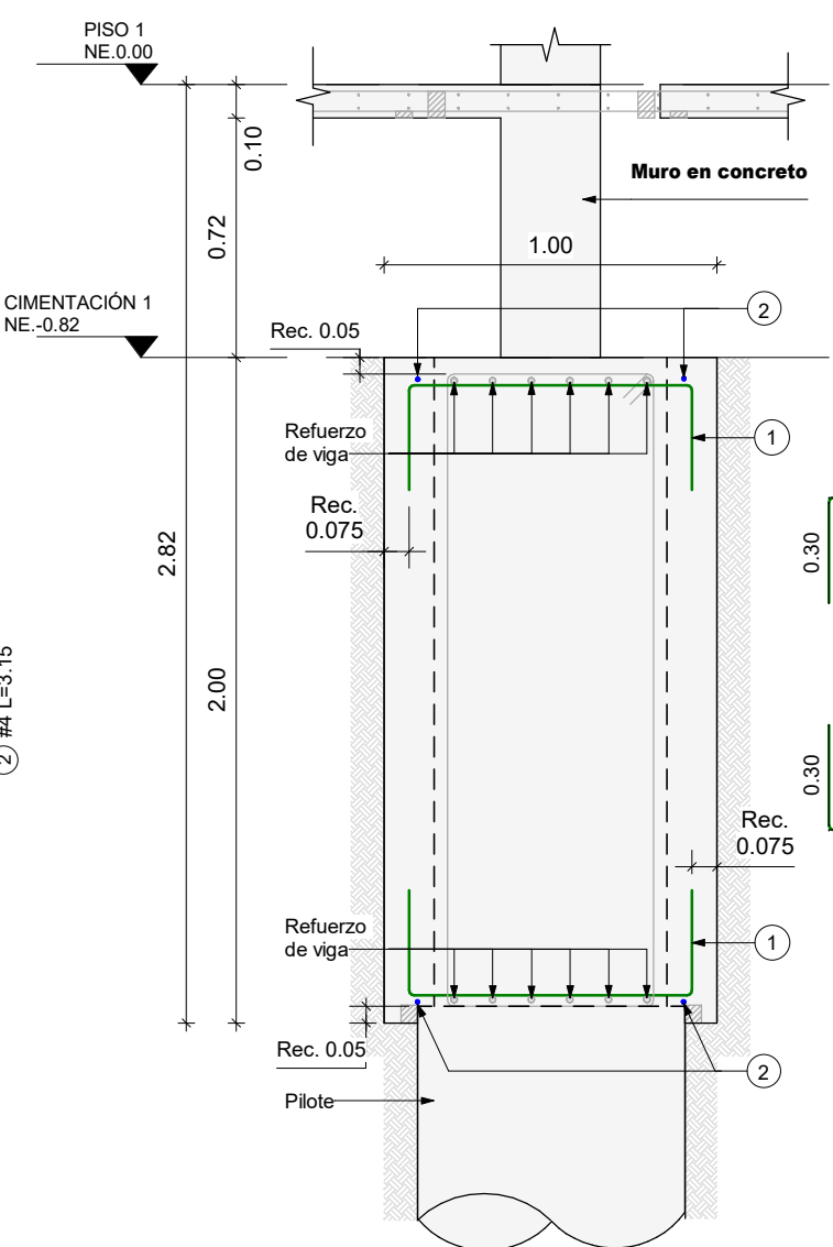
CORTE D2 Escala 1 : 25 DADO TIPO 1 Y 3
