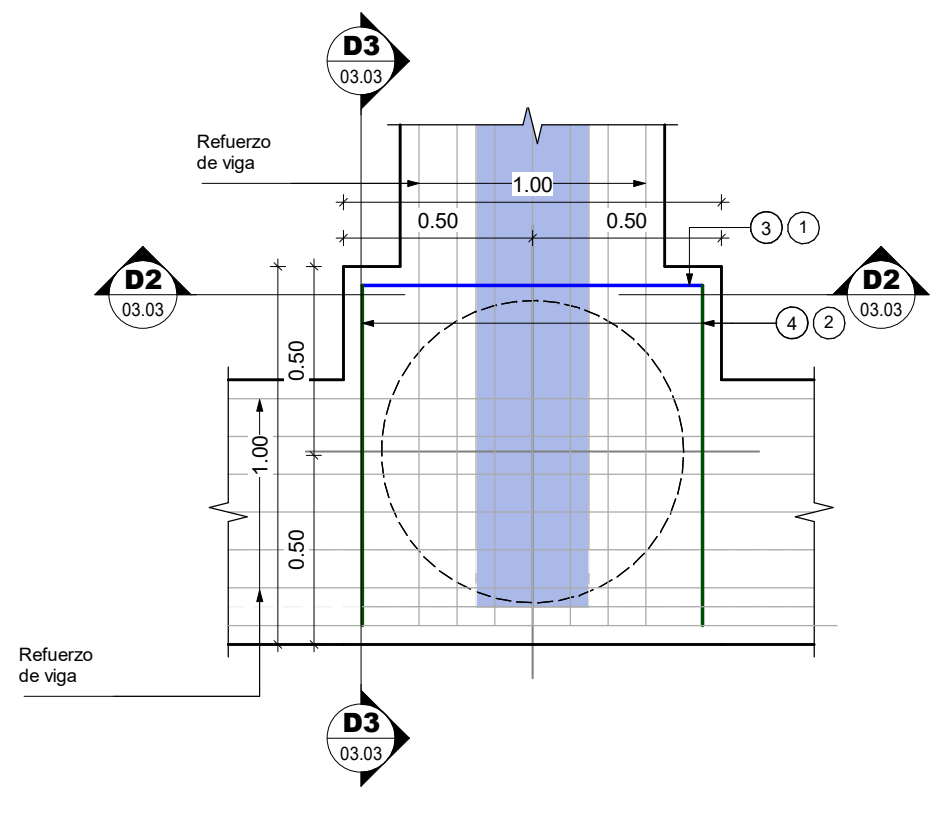
PLANTA REFUERZO TÍPICO DADOS TIPO 3 Y 4 Escala 1 : 20
