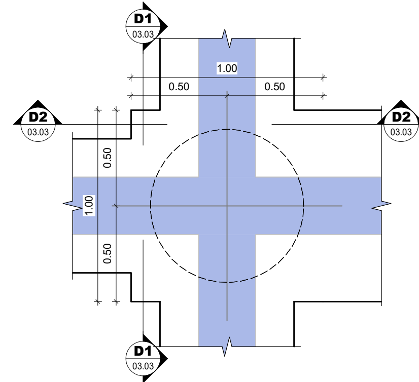
GEOMETRÍA TÍPICA DADOS TIPO 1 Y 2 Escala 1 : 20
