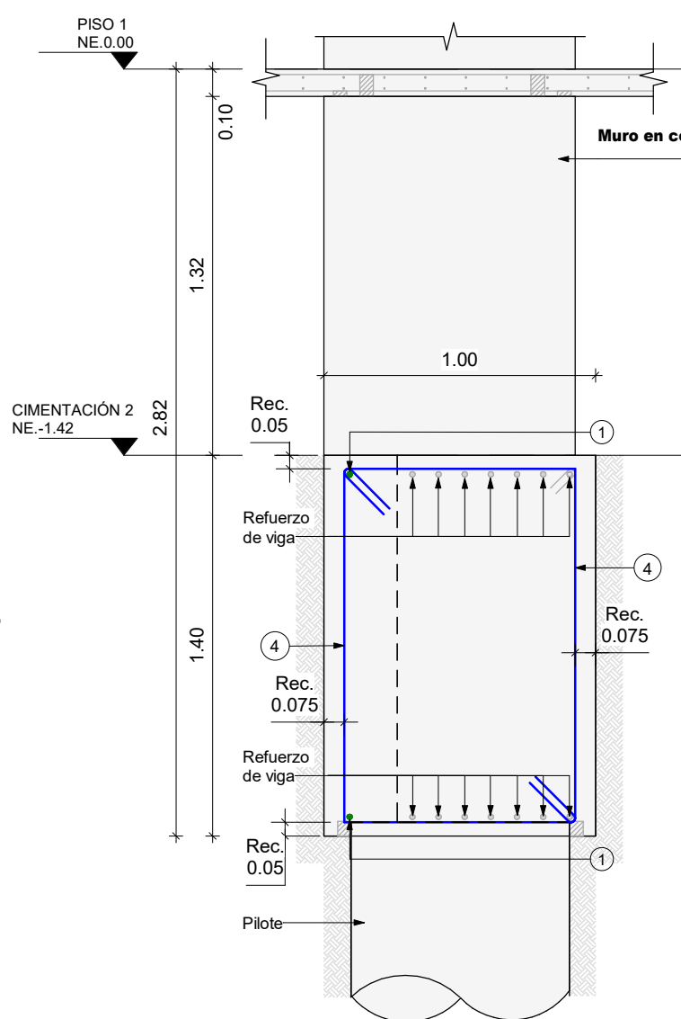
CORTE D4 Escala 1 : 25 DADO TIPO 4
