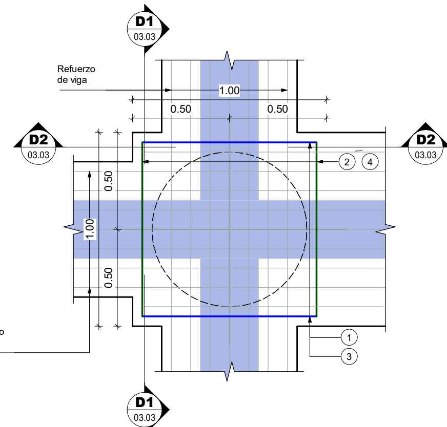
PLANTA REFUERZO TÍPICO DADOS TIPO 1 Y 2 Escala 1 : 20
