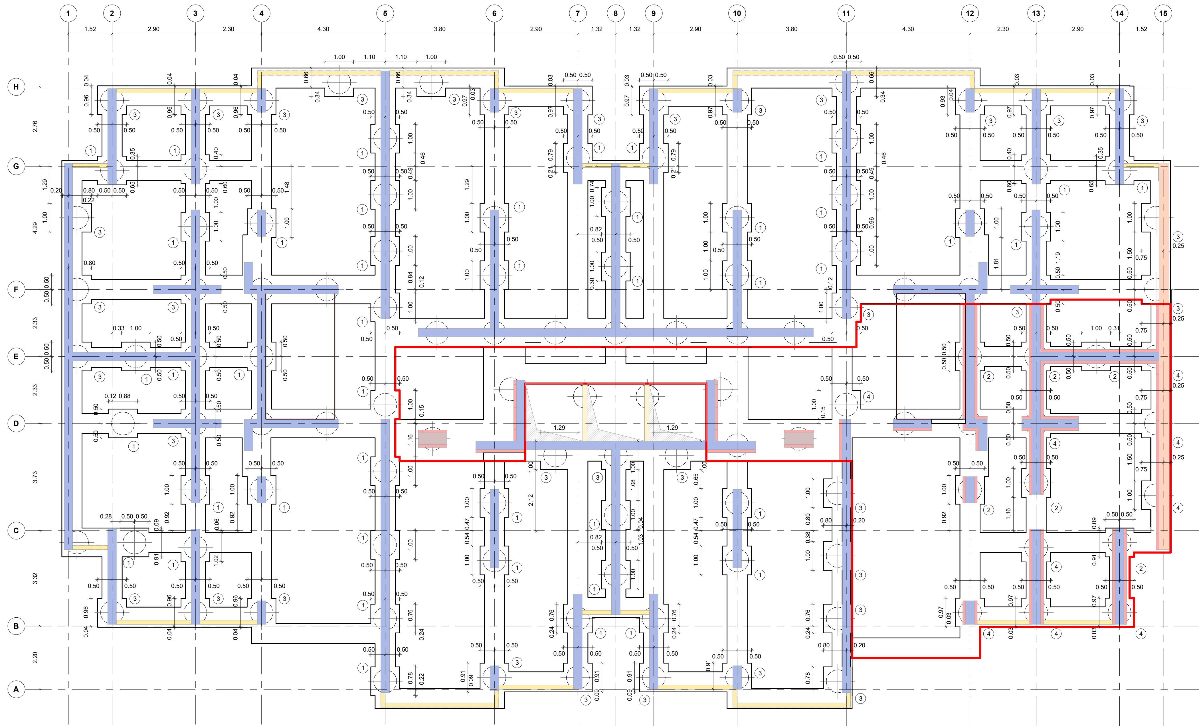
PLANTA DE LOCALIZACIÓN DE DADOS N.E -0.82 Y N.E -1.42 Escala 1 : 75
