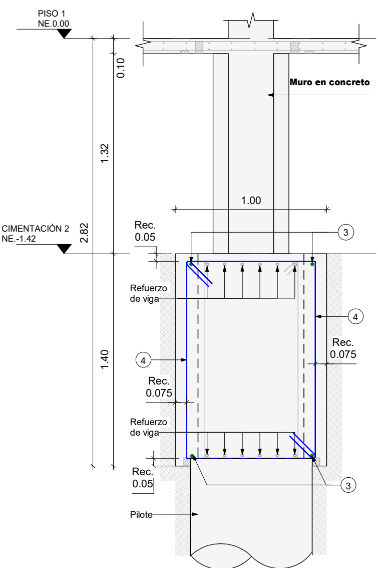
CORTE D1 Escala 1 : 25 DADO TIPO 2
